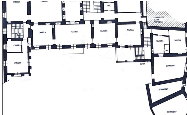
PIANO SOTTOTETTO scala 1:100
