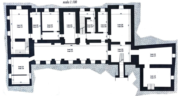
PIANO INTERRATO scala 1:100
