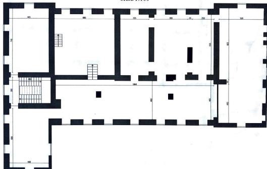
PIANO SOTTOTETTO scala 1:100
