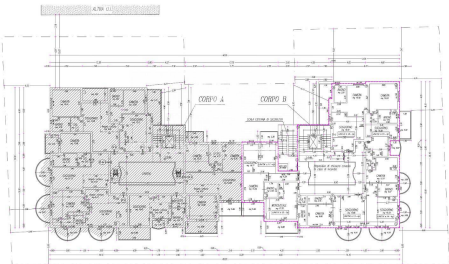
PIANTA PIANO 3°
