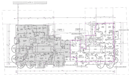
PIANTA PIANO 4°
