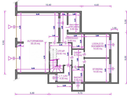
PIANTA PIANO INTERRATO
