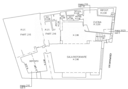
PIANO SOTTOSTRADA
