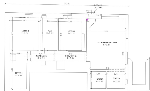
PIANTA PIANO SEMINTERRATO (CORPO A) DI PROGETTO SCALA 1:100
