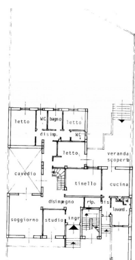
PIANO RIALZATO H. = 3,00
