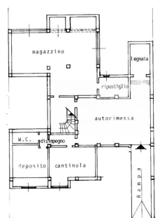
PIANO SEMINTERRATO H. = 3,00
