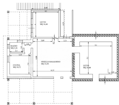
PIANTA
