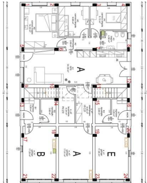
pianta piano terra - SX
