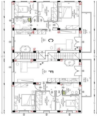
pianta piano primo - DX
