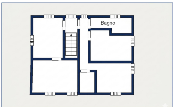
PIANO PRIMO
