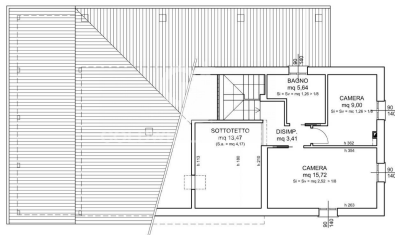
PIANO PRIMO scala 1:100
