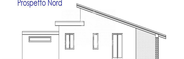
Prospetto Nord
