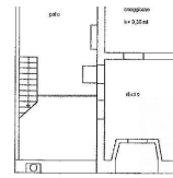
PIANTA PIANO TERRA
